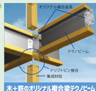
木+鉄のオリジナル複合梁テクノビーム
