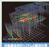
自動躯体設計システムの構造計算
