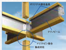
木+鉄のオリジナル複合梁テクノビーム
